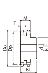
2列B形 削出仕様
