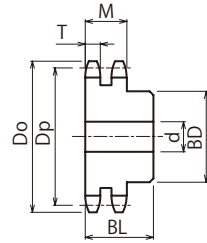
2列B形 削出仕様
