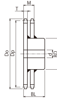
2列B形 溶接仕様
