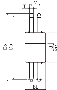
2列C形 溶接仕様
