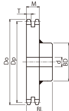
2列B形 溶接仕様
