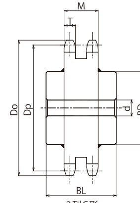
2列C形 溶接仕様
