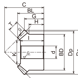
M3形状
