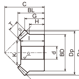
M3形状
