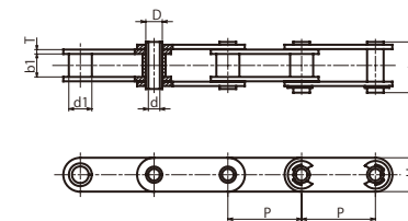
二バイピッチホローピンローラチェーン
