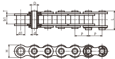
標準ホローピンローラチェーン
